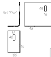
ANGOLARE PIEGATO A FREDDO
