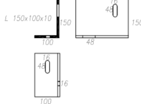
ANGOLARE LAMINATO A CALDO
