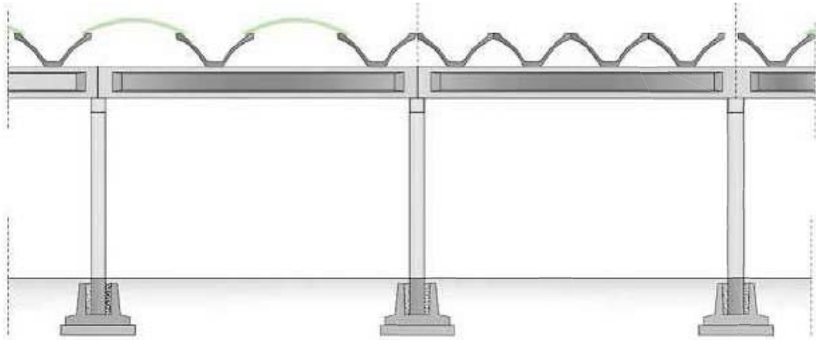
Figura 69 - Esempio di copertura realizzata con elementi speciali intervallati o meno da lucernari
