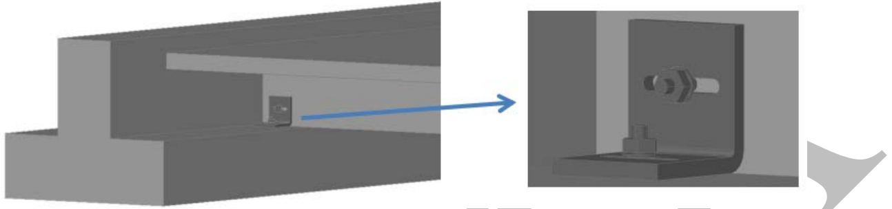
Figura 84 – Rinforzo connessione tegolo-trave: aggiunta di meccanismi di dissipazione con squadrette deformabili
